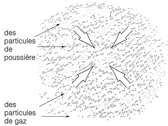
l'attraction gravitationnelle
