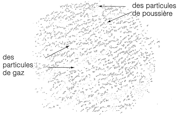
Une nébuleuse
